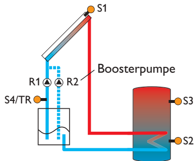
Beispielschema für ein Drainback-System (R2 = Boosterpumpe)
