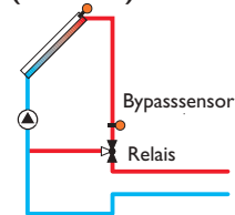
Variante Ventil (invertiert):
