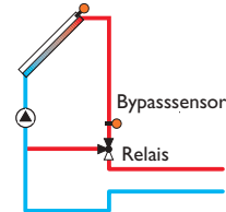
Variante Ventil:
